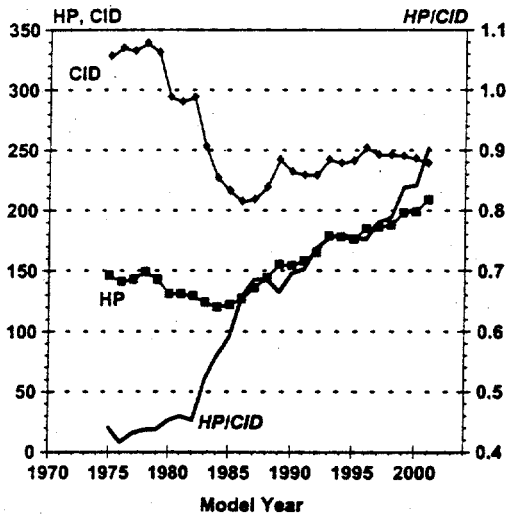
SUV Horsepower, CID and Horsepower per CID
